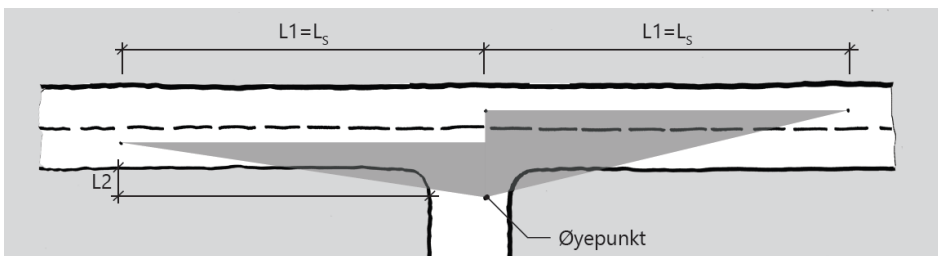
Figur 3: Siktretkant i avkjørsler (Kilde: N100, Vegdirektoratet)
